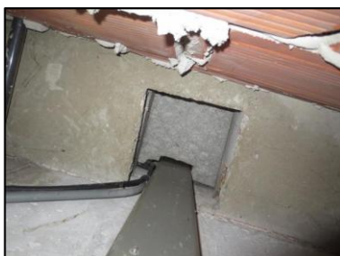
Photo N° 1141 AMIANTE CIMENT -- placards technique rdc à +6Planchers Plaques planes (Fibres- ciment)
